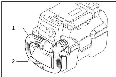
► 1. Hose 2. Hook
